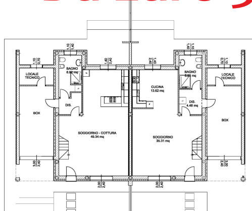
PIANTA PIANO TERRA SCALA: 1:100
